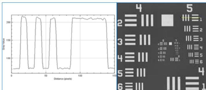
MTF 개선 동축 조명
