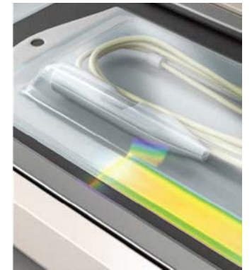
의료용 실타 무결성 검사
